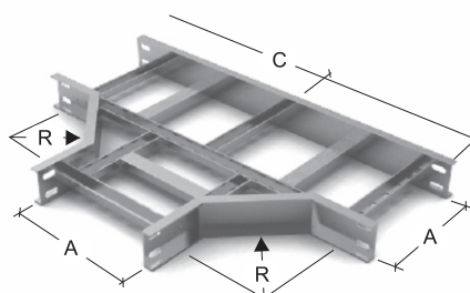
TÊ HORIZONTAL 90°
