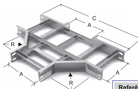
CRUZETA RETA C/ UMA SAÍDA RETA 90°
