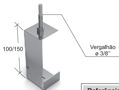
GANCHO CURTO E LONGO PARA PERFILADO
