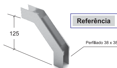
CURVA VERTICAL EXTERNA PARA PERFILADO
