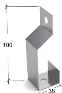
GANCHO J PARA CABO DE AÇO
