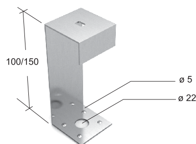
GANCHO CURTO E LONGO PARA LUMINÁRIA
