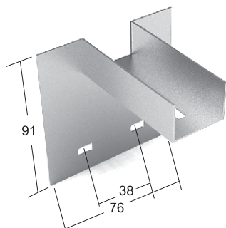
ACOPLAMENTO
