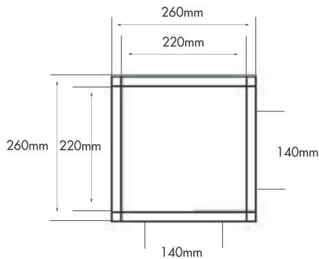
CAIXA QUADRADA 8X25X140MM COM TAMPA
