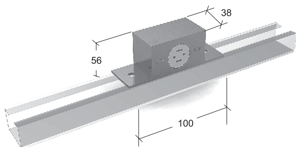
CAIXA PARA TOMADA
