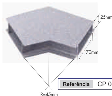
CURVA HORIZONTAL 45° PARA DUTO
