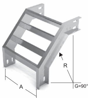
CURVA DE INVERSÃO
